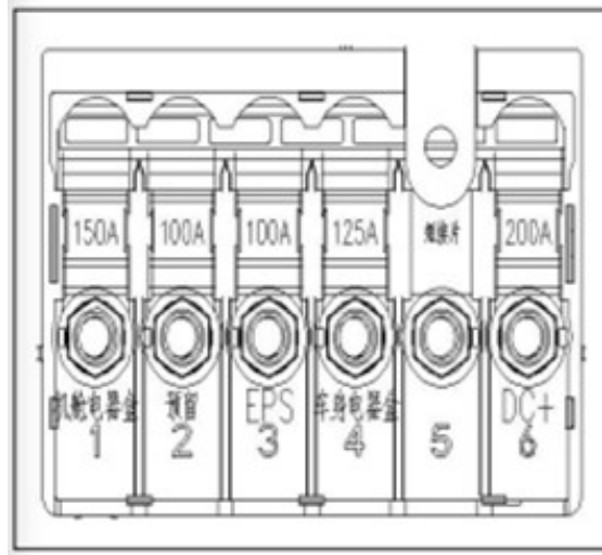
Corrente nominal e função do fusível na caixa de fusíveis do polo positivo da bateria.
